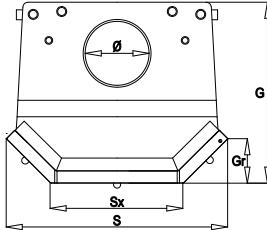
PL-190 Pryzma
